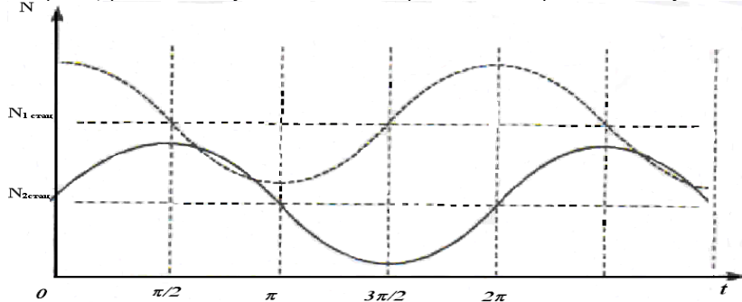
Рис 1. Зависимость изменения популяций от времени.
