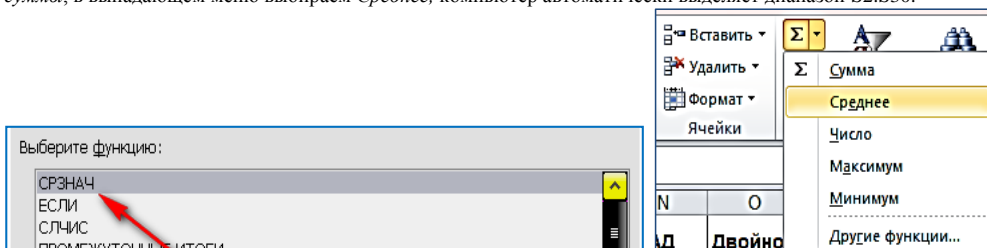
Рис. 22. Функция СРЗНАЧ
