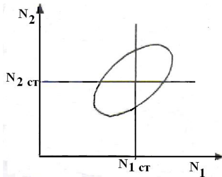
Рис 2. Графическая зависимость изменения численности популяций. Фазовый портрет системы.
